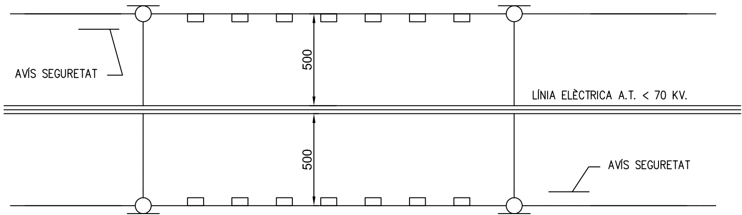
PLANTA ESCALA: 1/200
